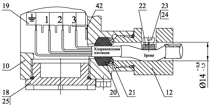
Рисунок 2.1 - Разделка и заделка конца кабеля
