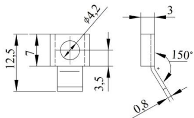
Шайба ТЖИУ.745522.002-03
