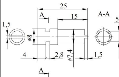
Ключ ТЖИУ.741131.057
