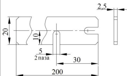
Ключ-пластина ТЖИУ.741131.056
